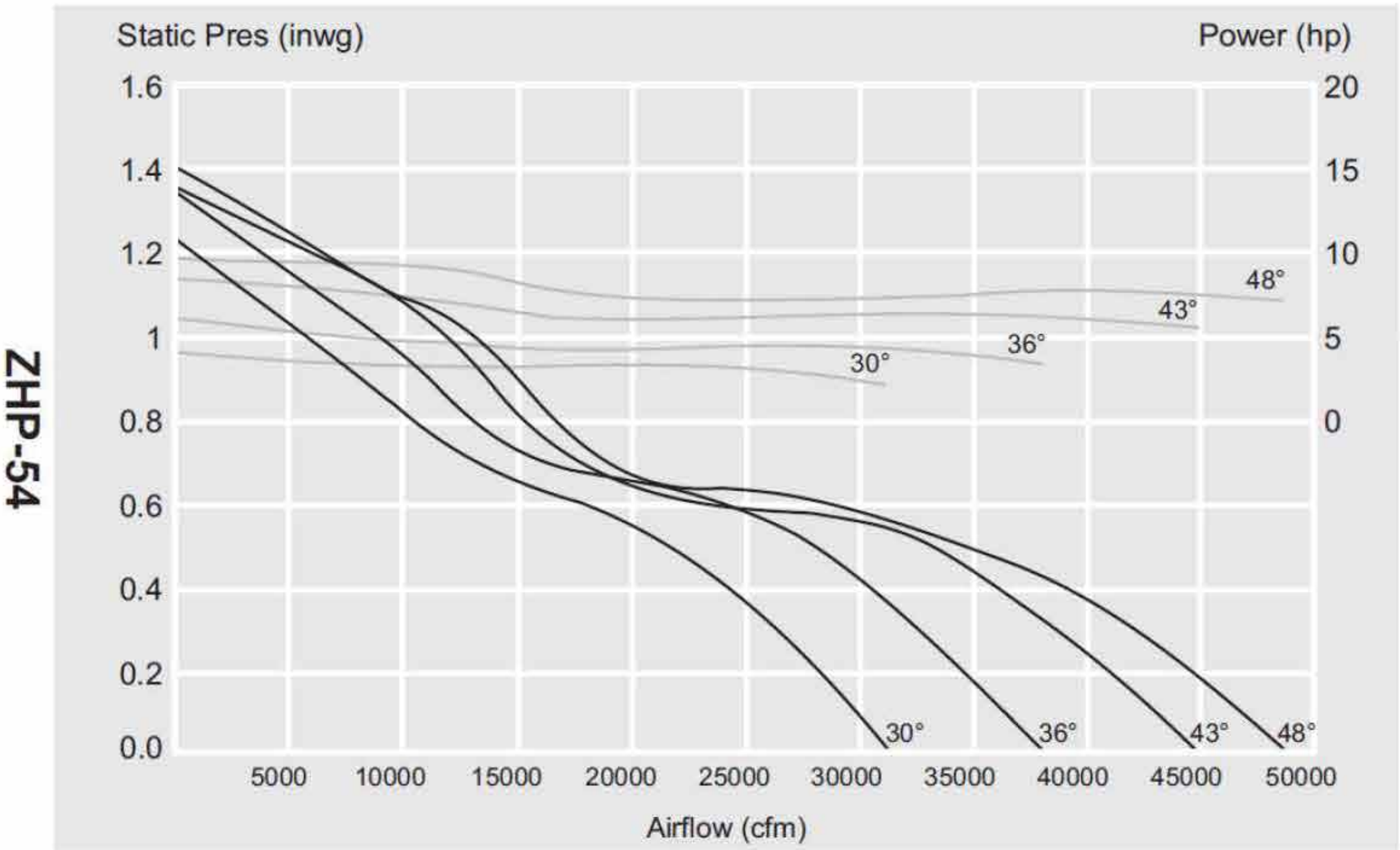
CURVAS DE OPERACIÓN (PERFORMANCE CURVES)
