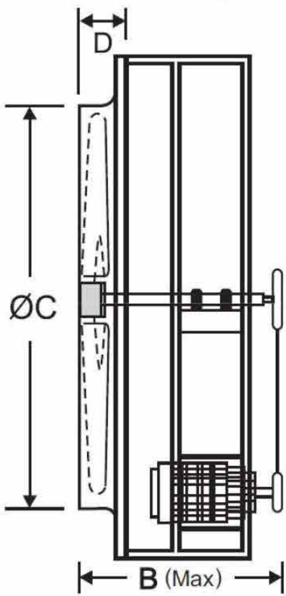
DIMENSIONES GENERALES (DIMENSIONS)
