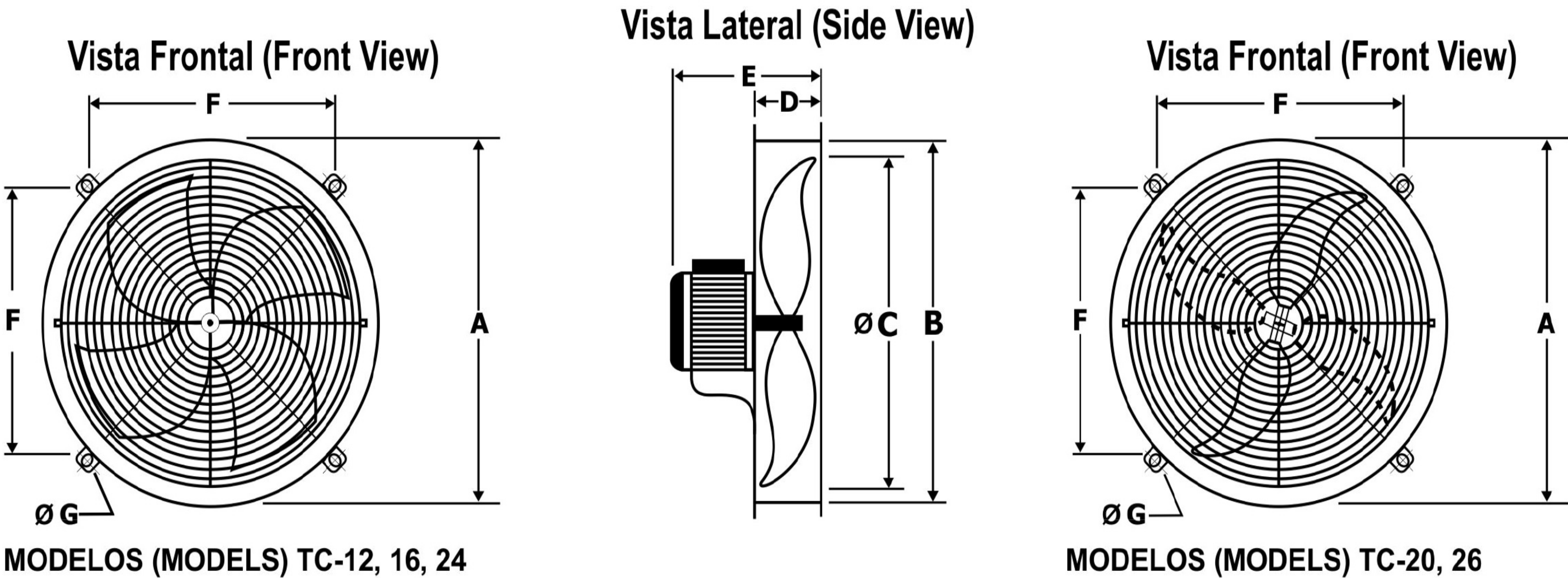
DIMENSIONES GENERALES (DIMENSIONS)
