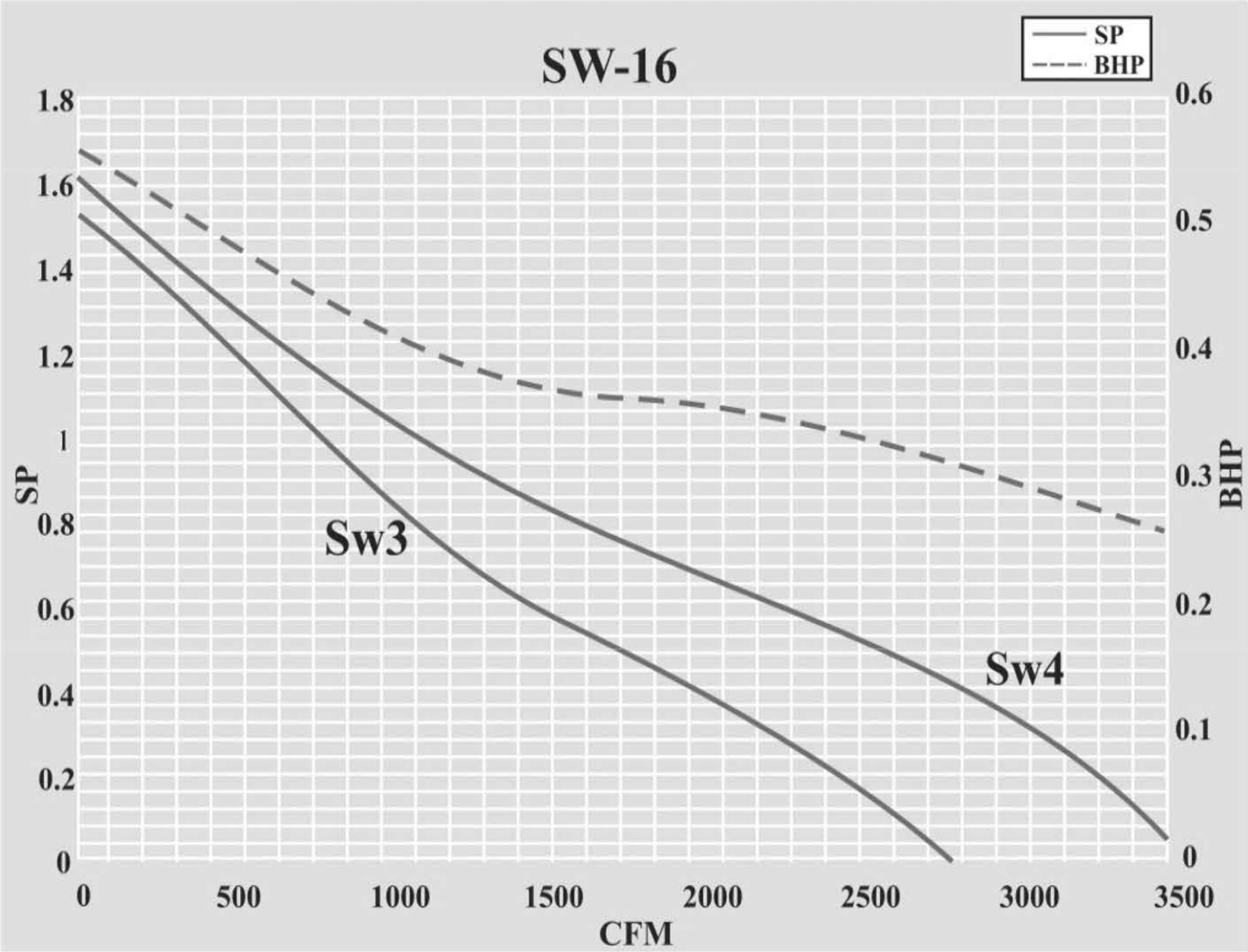
CURVAS DE OPERACIÓN (PERFORMANCE CURVES)
