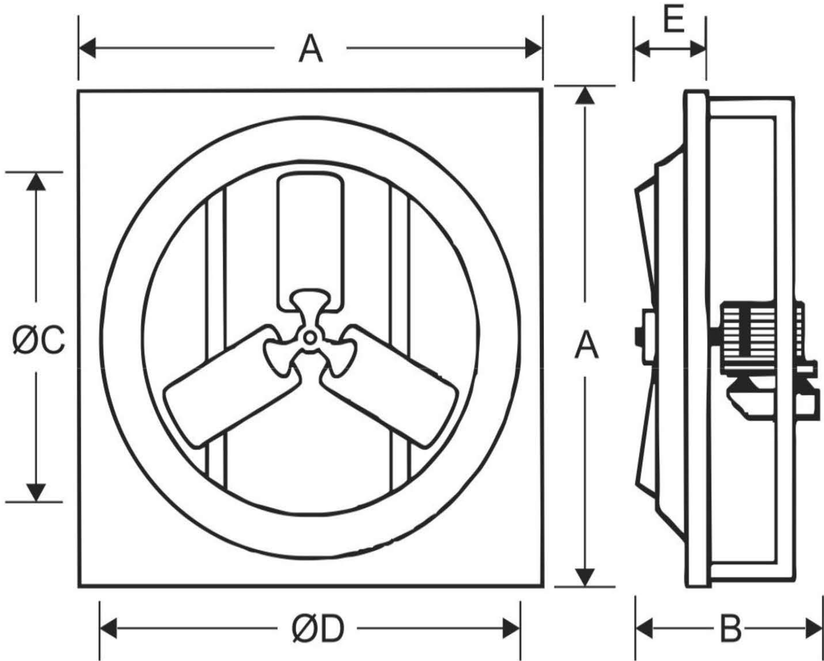
DIMENSIONES GENERALES (Dimensions)
