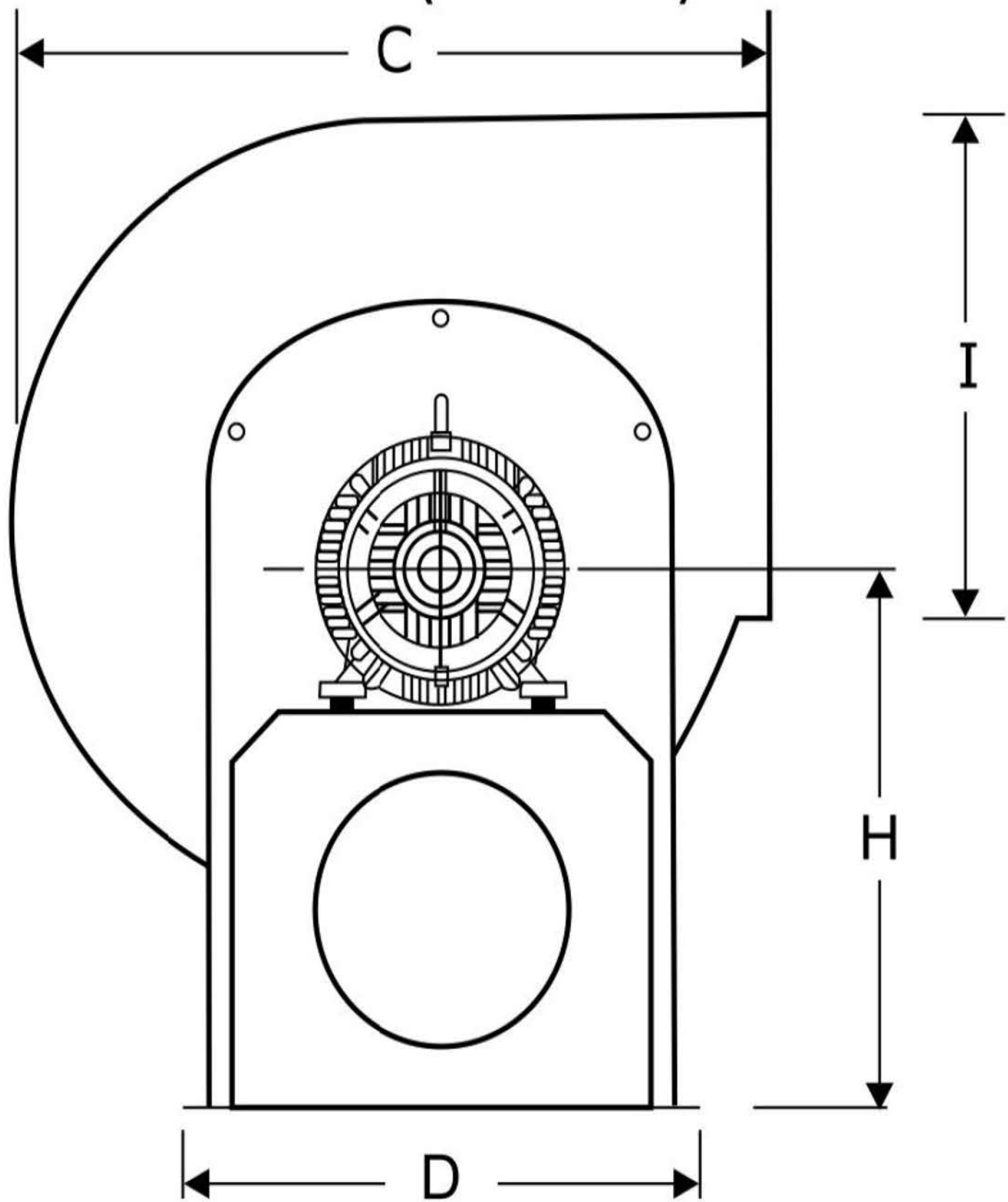
DIMENSIONES GENERALES (DIMENSIONS)
