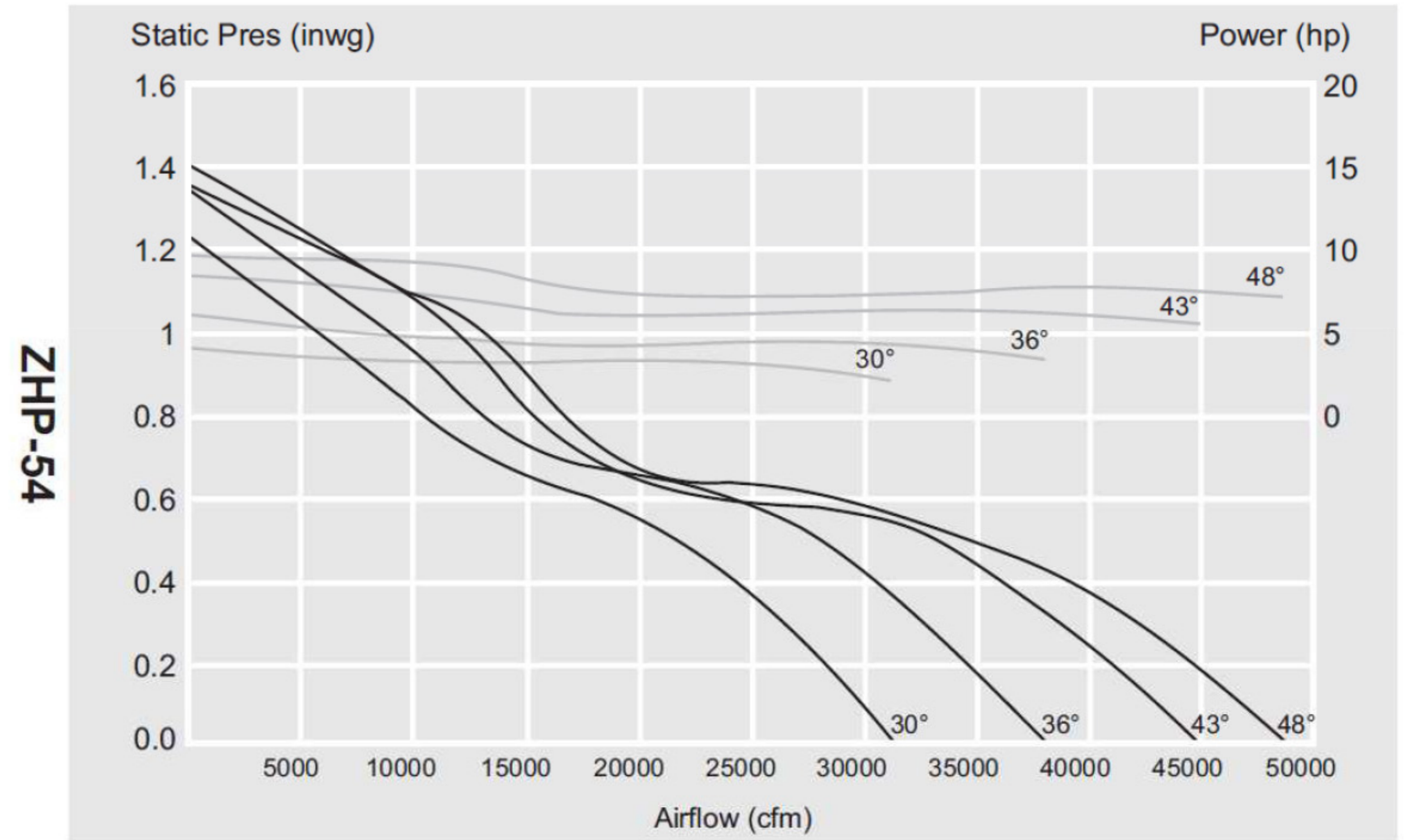
CURVAS DE OPERACIÓN (PERFORMANCE CURVES)
