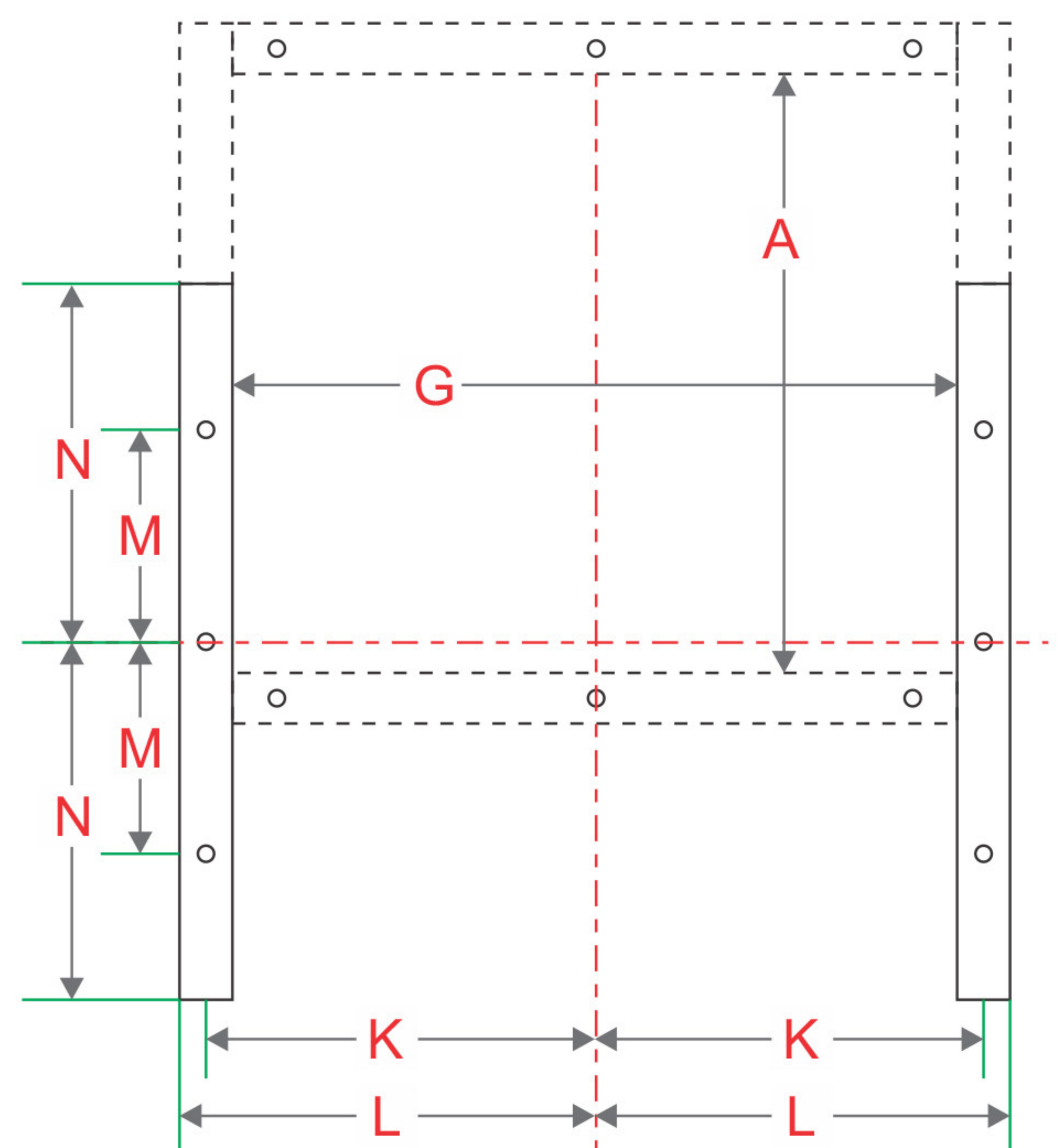
Vista planta para barrenos Foundation plan
