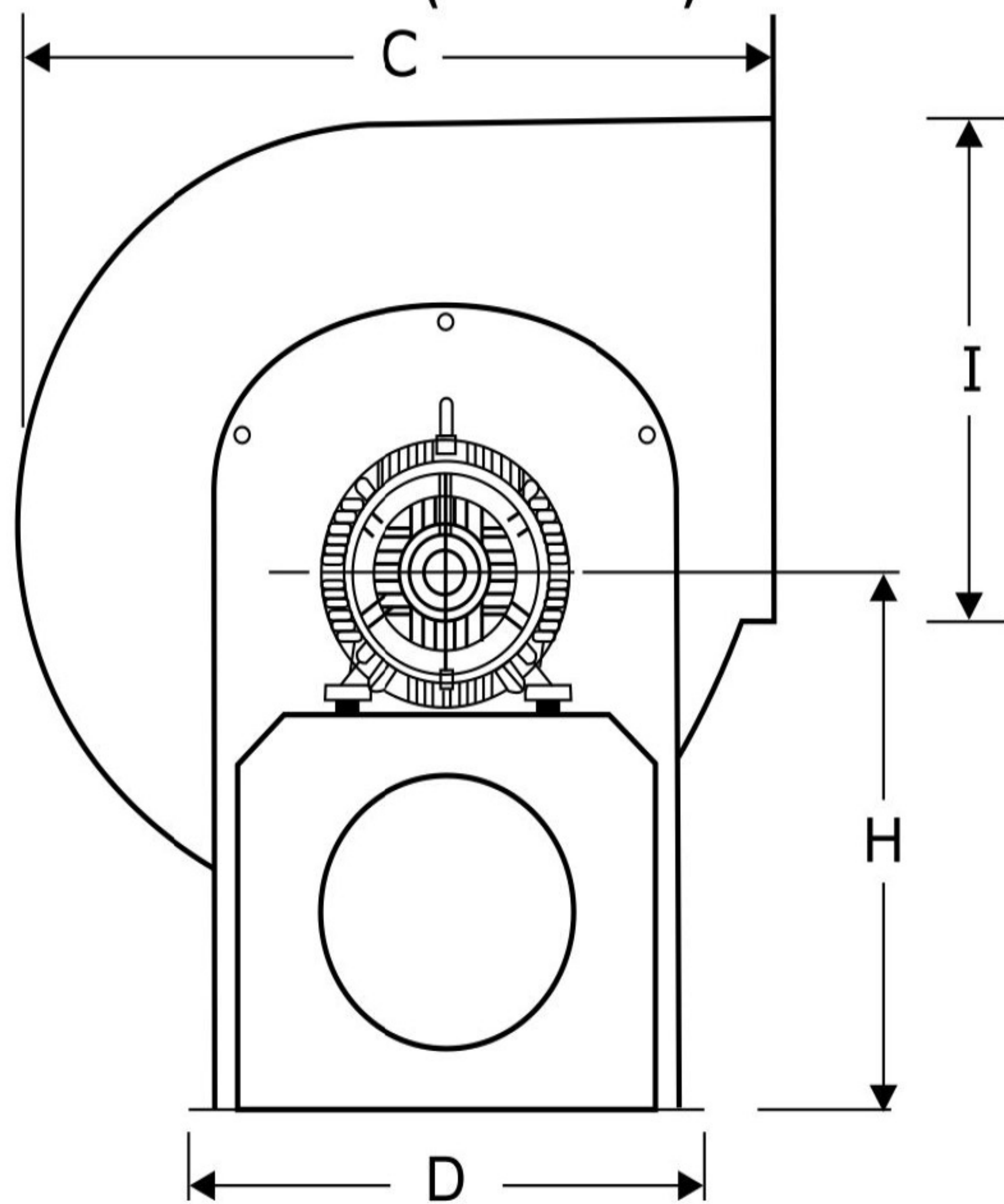
DIMENSIONES GENERALES (DIMENSIONS)
